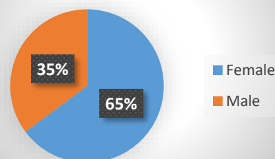
genderwise %
